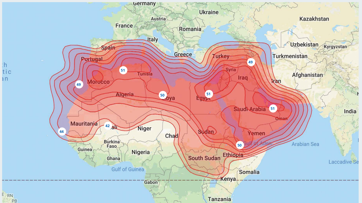
Footprint (EIRPs) dBW
