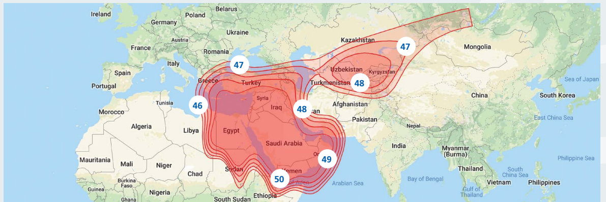
Footprint (EIRPs) dBW
