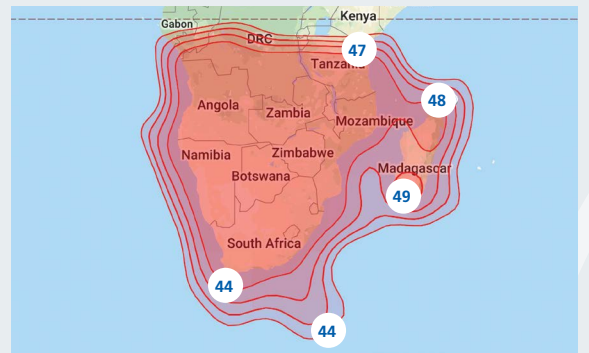
Footprint (EIRPs) dBW
