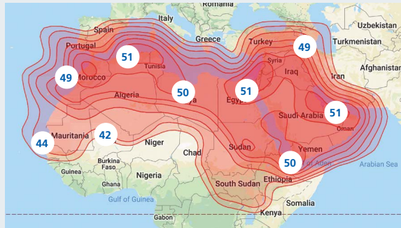
Footprint (EIRPs) dBW
