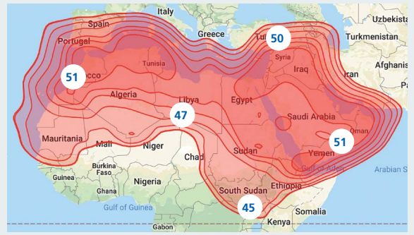
Footprint (EIRPs) dBW
